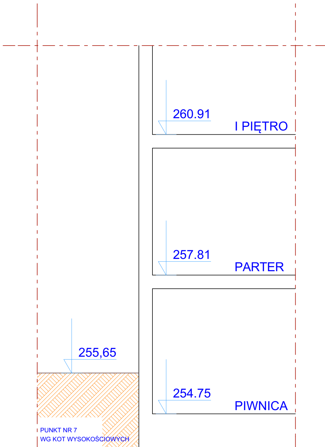
SCHEMAT PRZEKROJU ISTNIEJĄCEGO BUDYNKU SZKOŁY MUZYCZNEJ W JASTRZĘBIU ZDROJU
