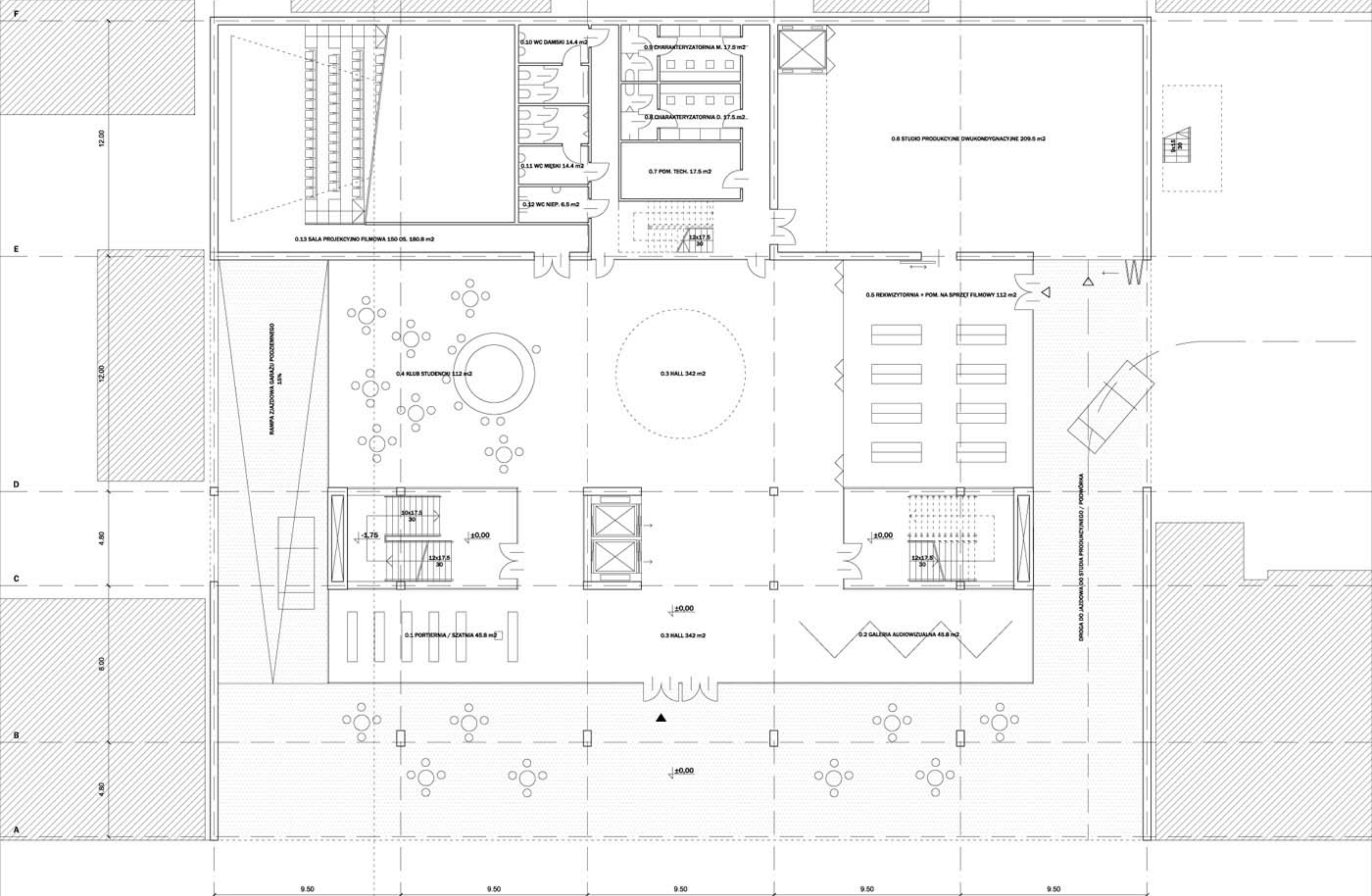
KONDYGNACJA 0 (PRZYZIEMIE) SKALA 1:100
