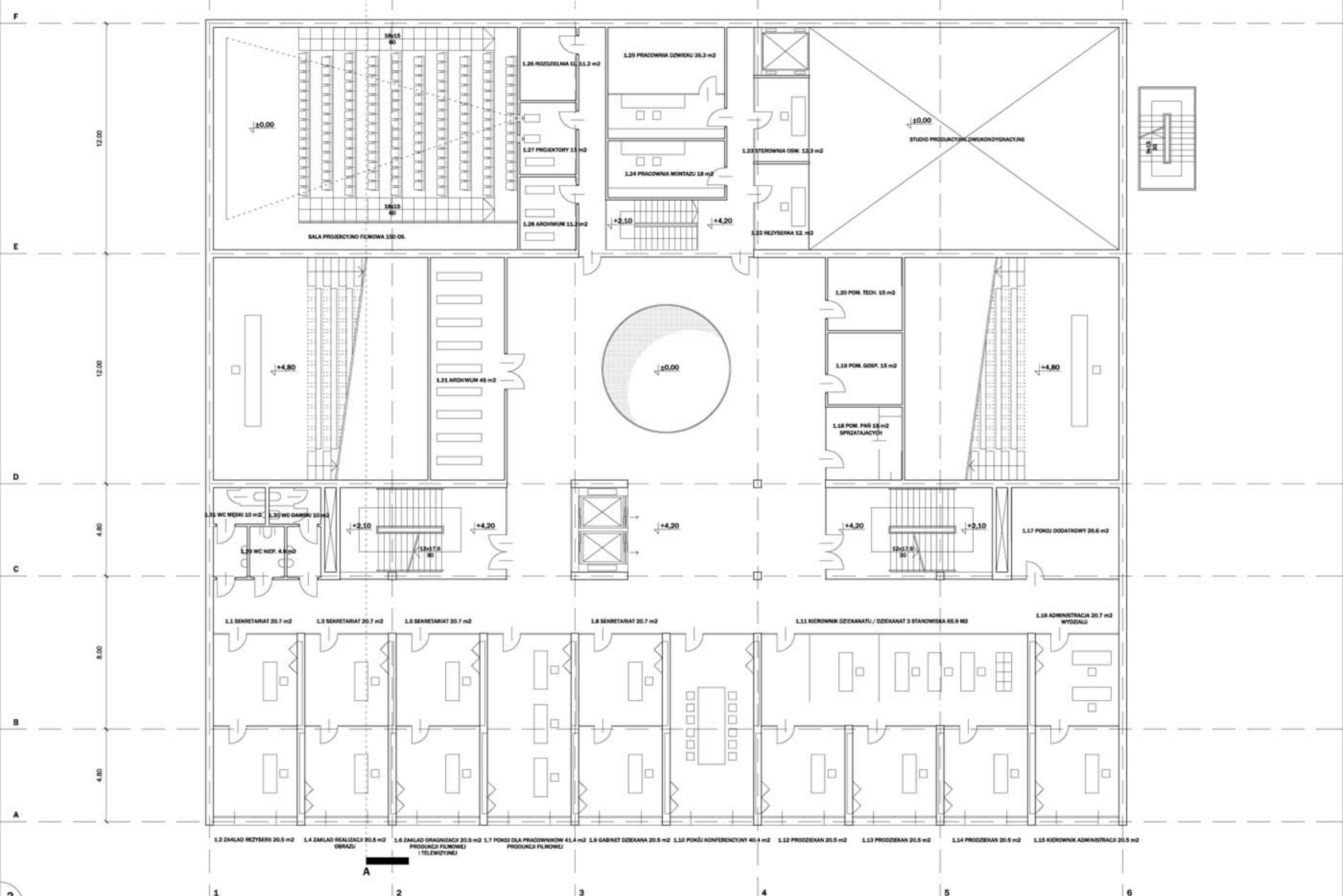
KONDYGNACJA +1 SKALA 1:100
