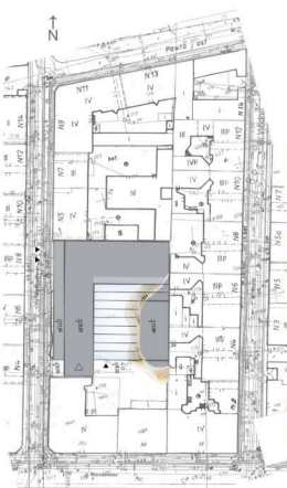
ZAGOSPODAROWANIE TERENU
